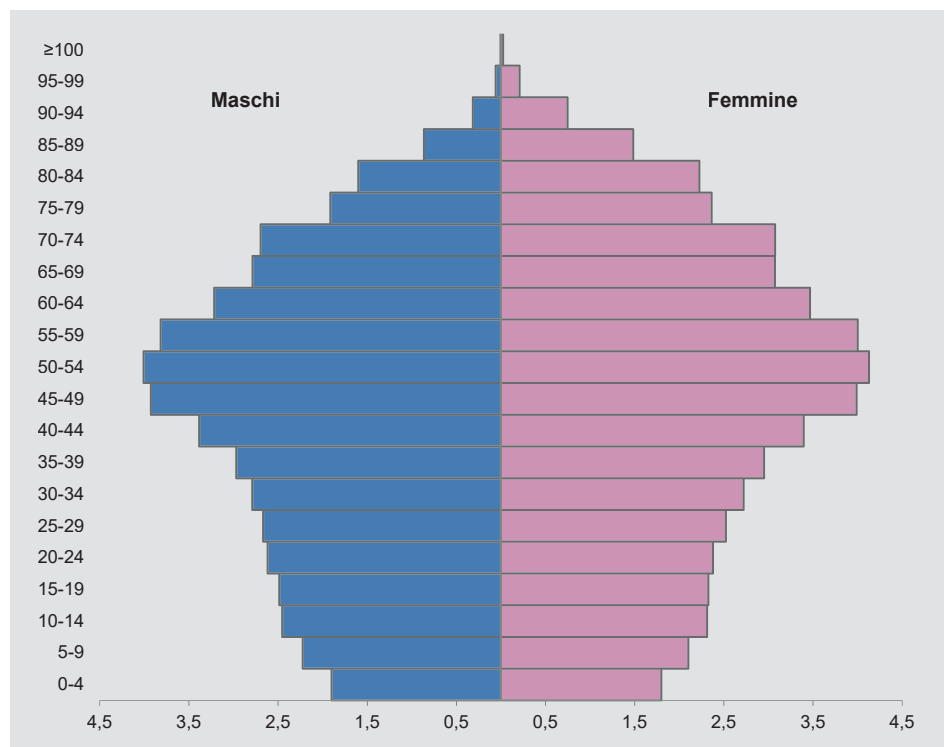
Figura 3.2 Piramide dell'età della popolazione residente per età e sesso al 1° gennaio Anno 2021, valori percentuali
